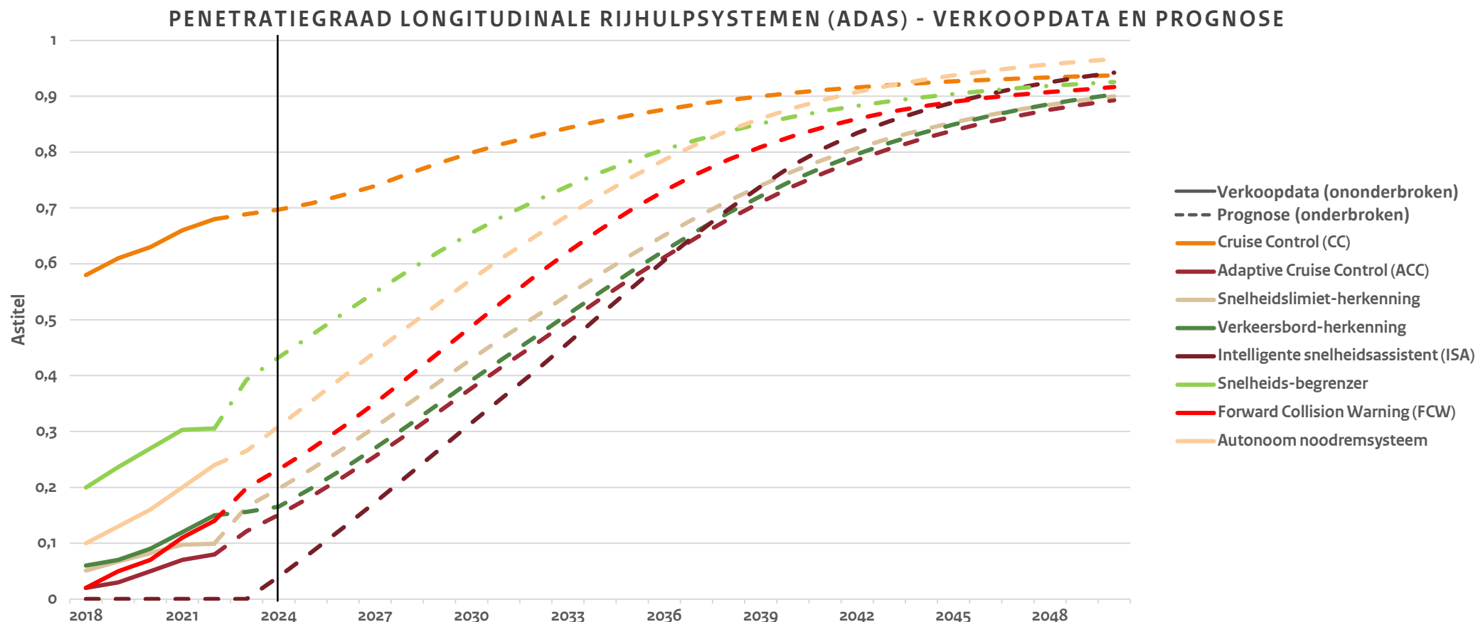
Figuur 3– Ingroei longitudinale rijhulpsystemen (ADAS) – gecombineerde verkoopdata VMS insights en prognose 3,4
